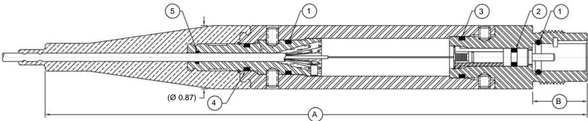
SECTION A-A
